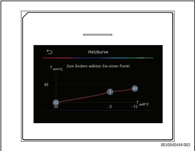
Bild 1 Startbildschirm für die Einstellung der Heizkurve für die Regelungsart Außentemperatur mit Fußpunkt (und Komfortpunkt)
