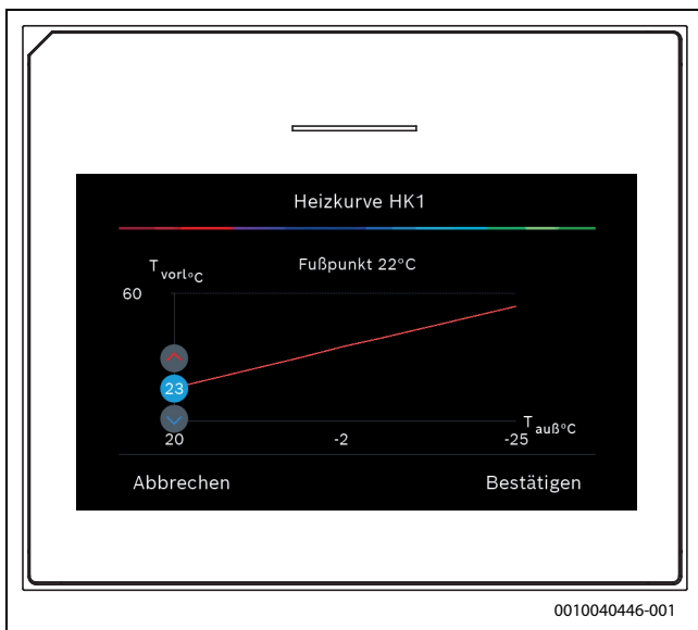
Bild 3 Fußpunkt einstellen
