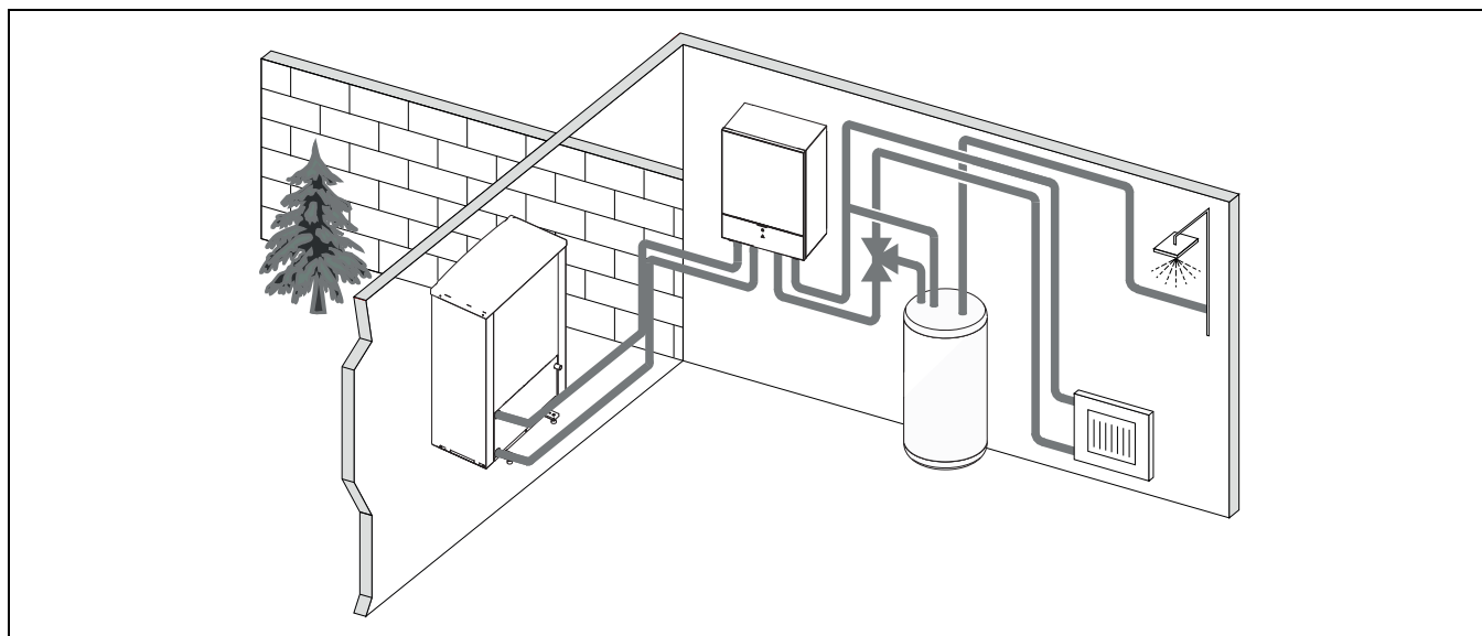
Fig. 3 Pompa di calore Compress 7000i AW unità interna AWE con riscaldatore elettrico supplementare e accumulatore-produttore d'acqua calda sanitaria esterno
