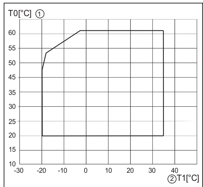
Fig. 1 Pompa di calore senza generatore di calore supplementare
