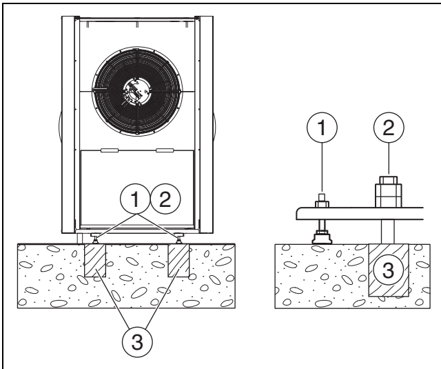
Fig. 14 Fixation de la pompe à chaleur
