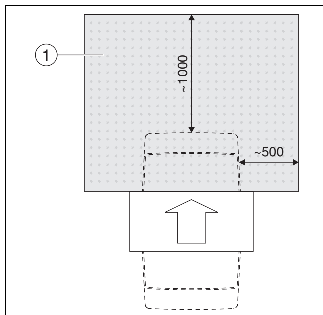
Fig. 11 DANGER ! Formation de glace devant les pompes à chaleur avec dispositif antibruit (accessoire)
