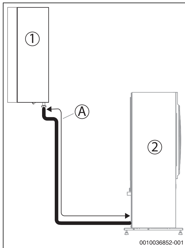
Fig. 16 Longueur du tuyau A
