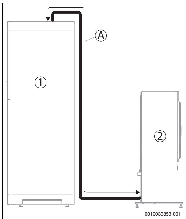
Fig. 15 Longueur du tuyau A
