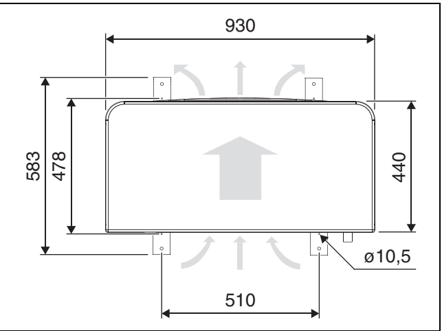
Fig. 5 Dimensions des modèles de pompe à chaleur 5 OR-S-9 OR-S, vue du dessus
