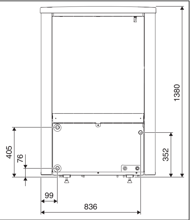
Fig. 4 Dimensions et raccords des modèles de pompe à chaleur 5 OR-S-9 OR-S, partie arrière
