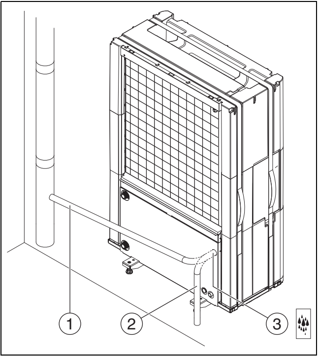
Fig. 17 Raccordements de tube de condensats, valable pour toutes les tailles
