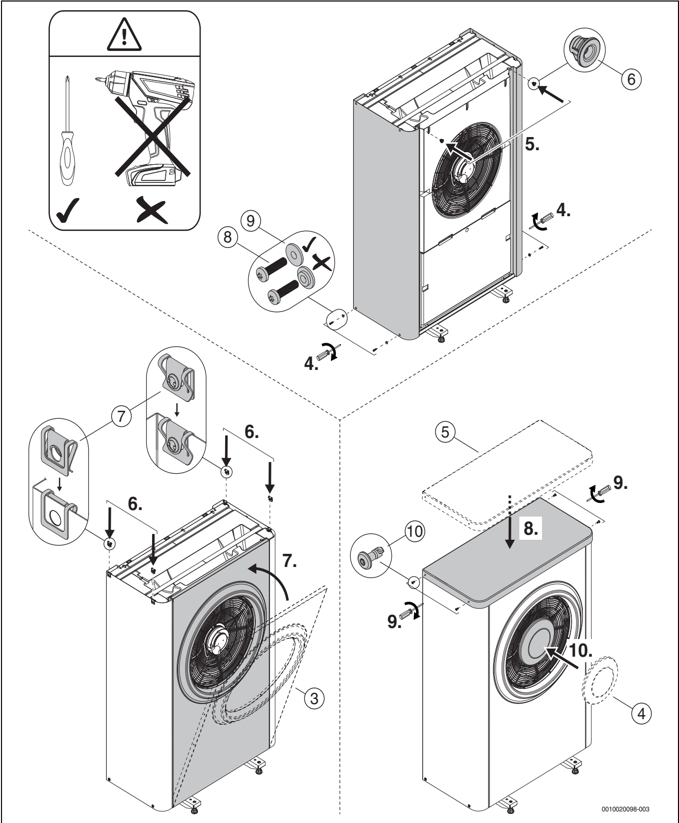
Fig. 22 Monter le couvercle et tôles latérales
