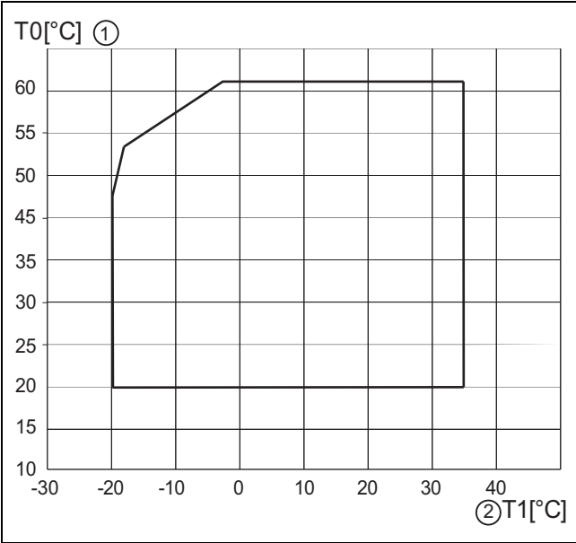
Fig. 23 Pompe à chaleur sans chauffage d'appoint
