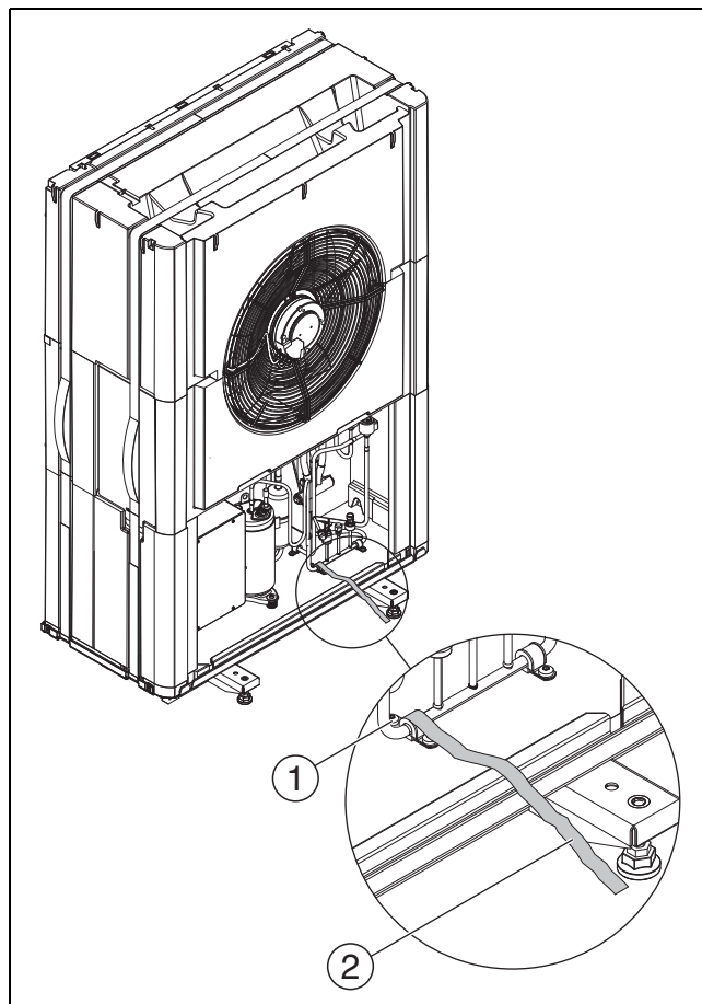
Fig. 13 Sécurisation pour le transport
