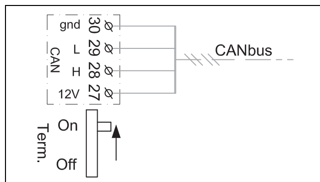
Fig. 19 Terminaison CAN-BUS
