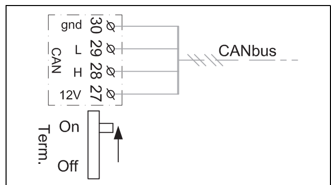
Bild 18 CAN-BUS-Terminierung
