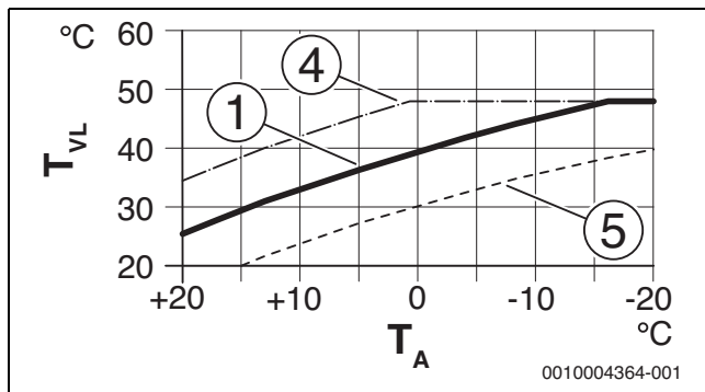
Fig. 6 Spostamento parallelo di una curva termocaratteristica di riscaldamento per mezzo del Offset temp. locale o della temperatura aria ambiente richiesta
