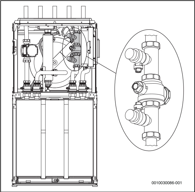
Bild 27 Befüllereinrichtung
