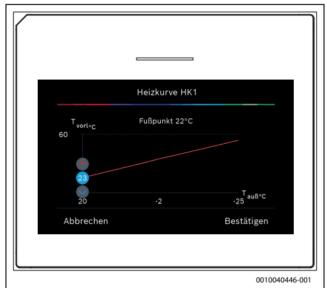
Bild 3 Fußpunkt einstellen
