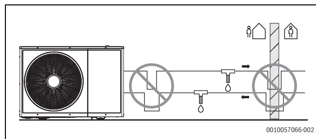
Fig. 22 Installation de la vanne antigel
