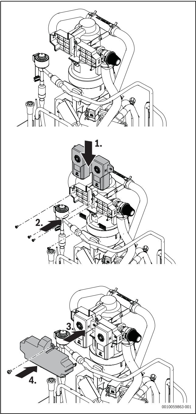
Fig. 45 Remplacement des capteurs R290
