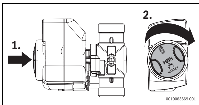
Fig. 42 Fonctionnement manuel de la vanne normalement fermée
