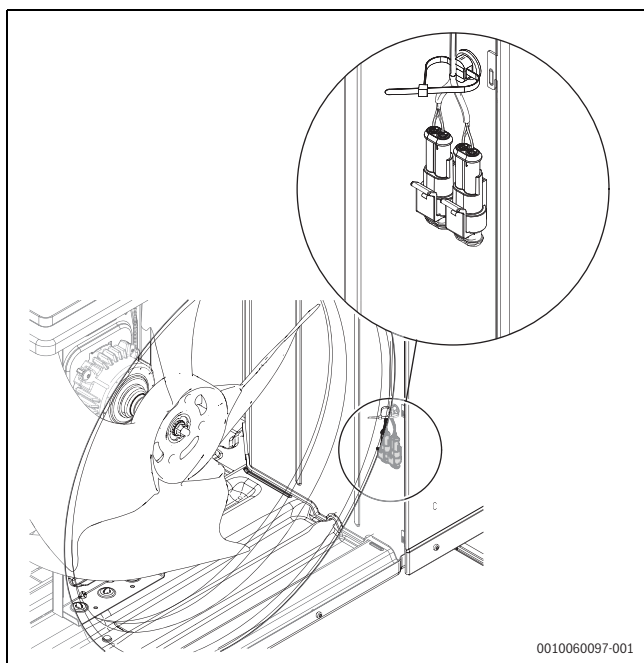
Fig. 39 Élément chauffant du bac de récupération et raccordement du câble de chauffage
