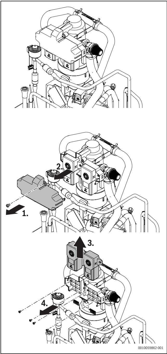
Fig. 44 Remplacement des capteurs R290
