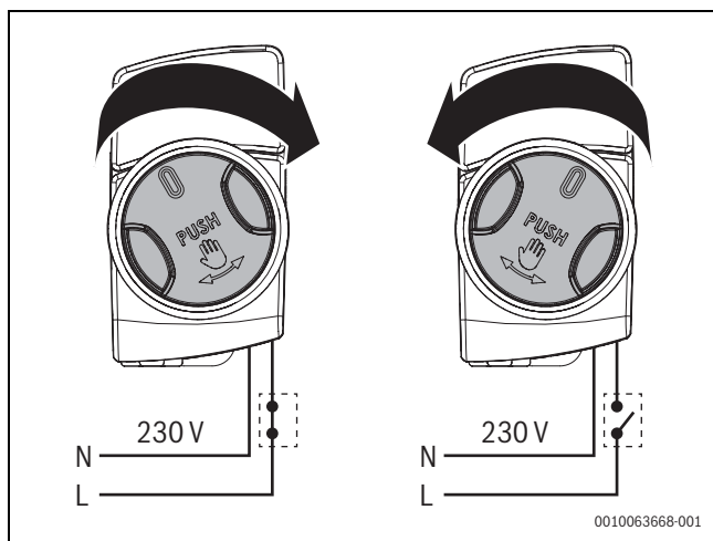
Fig. 41 Principe de fonctionnement de la vanne normalement fermée
