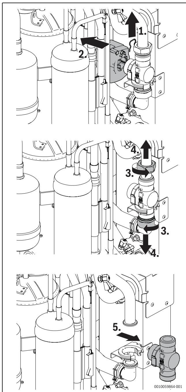
Fig. 46 Remplacement de tuyaux NCV
