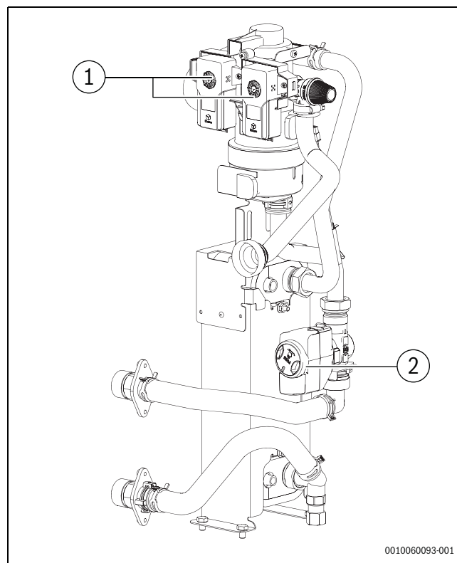
Fig. 43 Kit de sécurité propane
