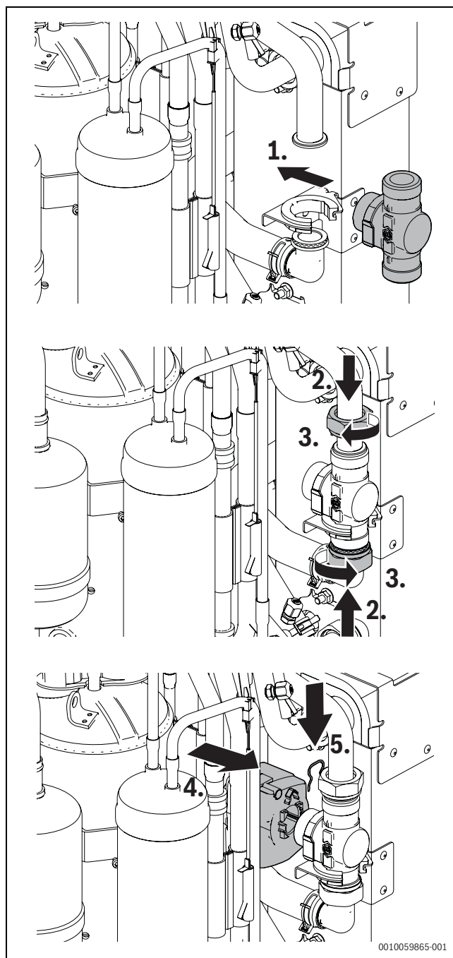
Fig. 47 Remplacement de tuyaux NCV
